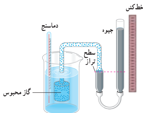
شکل ۴-۴۵ آزمایشی ساده برای اندازه گیری فشار گاز در دماهای مختلف (در حجم ثابت)
