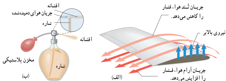
شکل ۳-۳۱- ب کاربرد اصل برنولی در الف) بال هواپیما برای ایجاد نیروی بالابر
