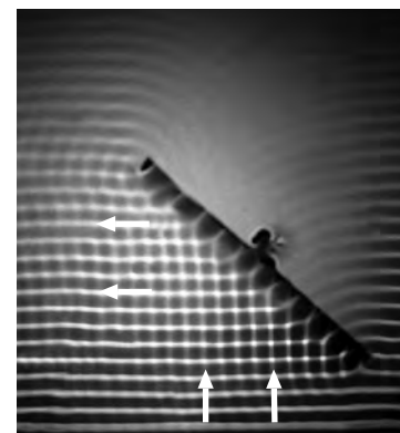
شکل ۳-۳۴ بازتاب امواج تخت از مانع تخت در تشت موج.
